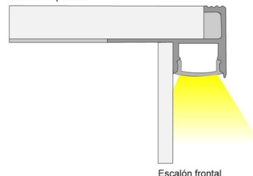
Escalón superficie
