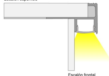
Escalón frontal
