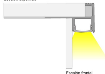
Escalón superficie
